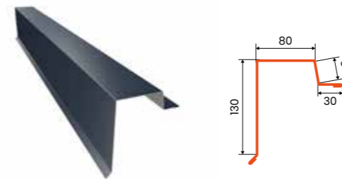
PHR Ortgangblech/Dachrandprofil
