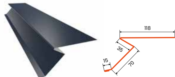
PHR Traufenblech / Rinneneinhangblech
