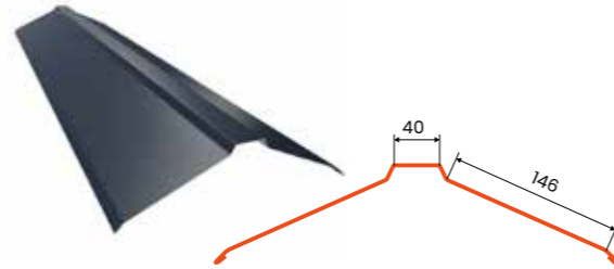
PHR trapezförmiger Streifen
