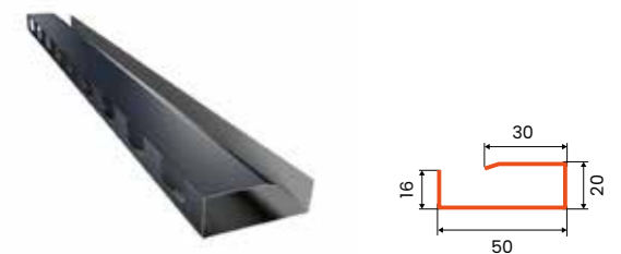
PHR Unterfirstleiste
