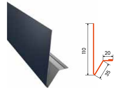
Speziell Unteres Traufblech
