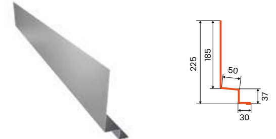
Seitenverbindungsteil PHR
