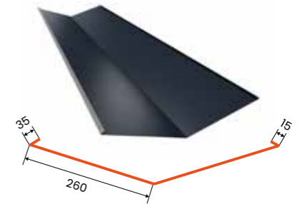
PHR Kehlrinne
