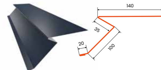
Trapezförmige Traufenblech / Rinneneinhangblech gross
